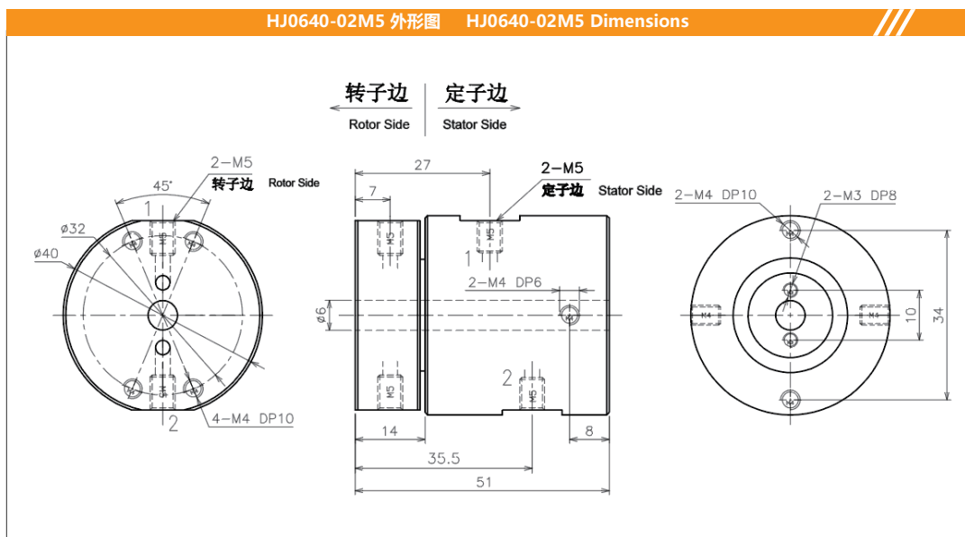
接口(M5)标准系列外形图
