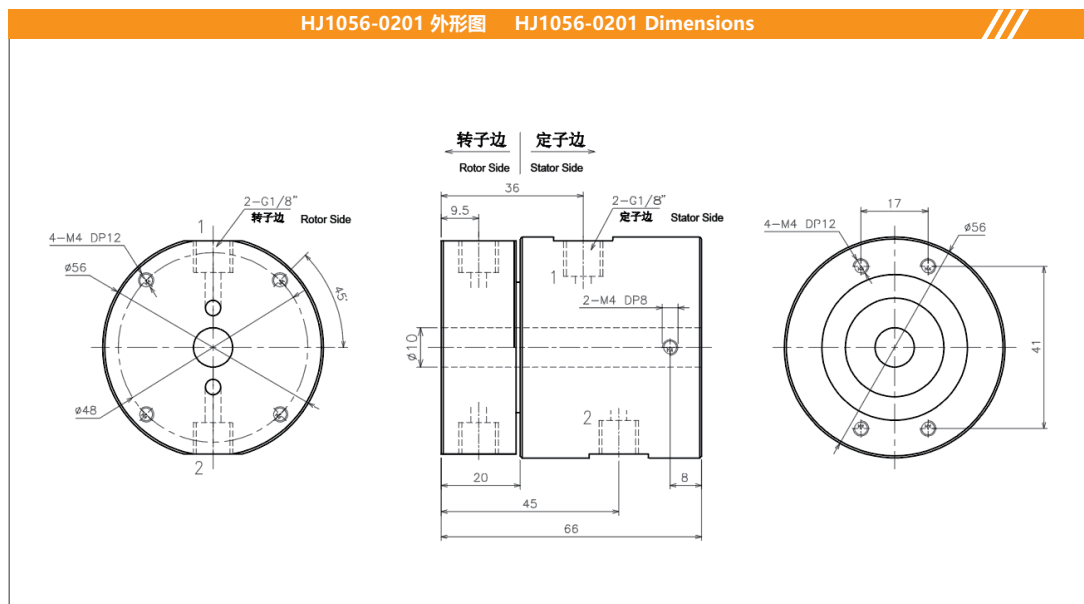
接口(G1/8)标准系列外形图
